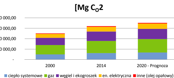
Emisja generowana przez pokrycie zapotrzebowania na energię cieplną
